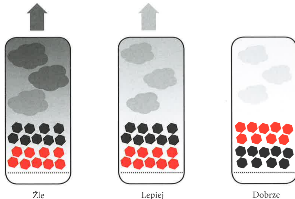
Rys. 12. Sposób spalania dolny vs górny
