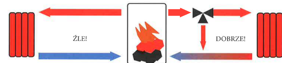
Rys. 13. Zastosowanie zaworu mieszającego
